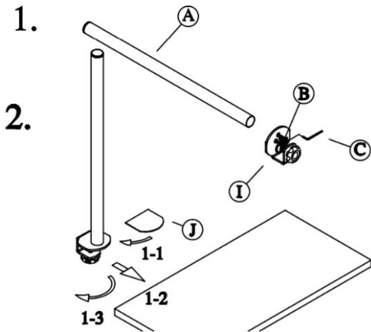
OPTION A./ Clamp to Edge
